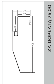
ościeżnica PD56/150
