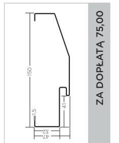
ościeżnica PD56/150
