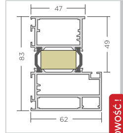
ościeżnica Termo ALU 68
