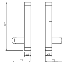
KLAMKA LEWA DO DRZWI LEWYCH OTWIERANYCH NA ZEWNĄTRZ I PRAWYCH OTWIERANYCH DO WEWNĄTRZ
