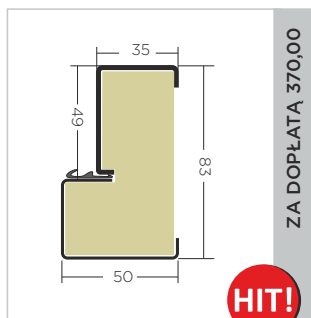
ościeżnica Termo ODS68
