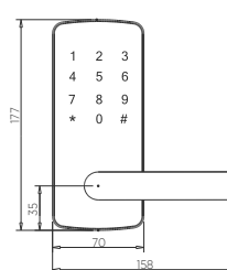
KLAMKA PRAWA DO DRZWI PRAWYCH OTWIERANYCH NA ZEWNĄTRZ I LEWYCH OTWIERANYCH DO WEWNĄTRZ
