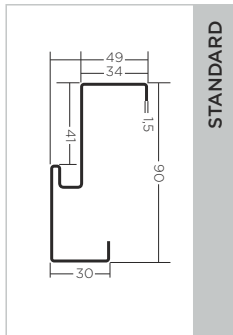
ościeżnica PU56
